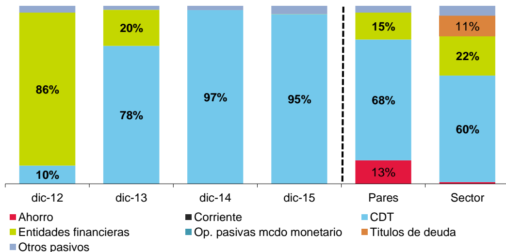
Gráfico 4 Composición del pasivo de Credifinanciera frente a los pares y el sector de compañías de financiamiento
