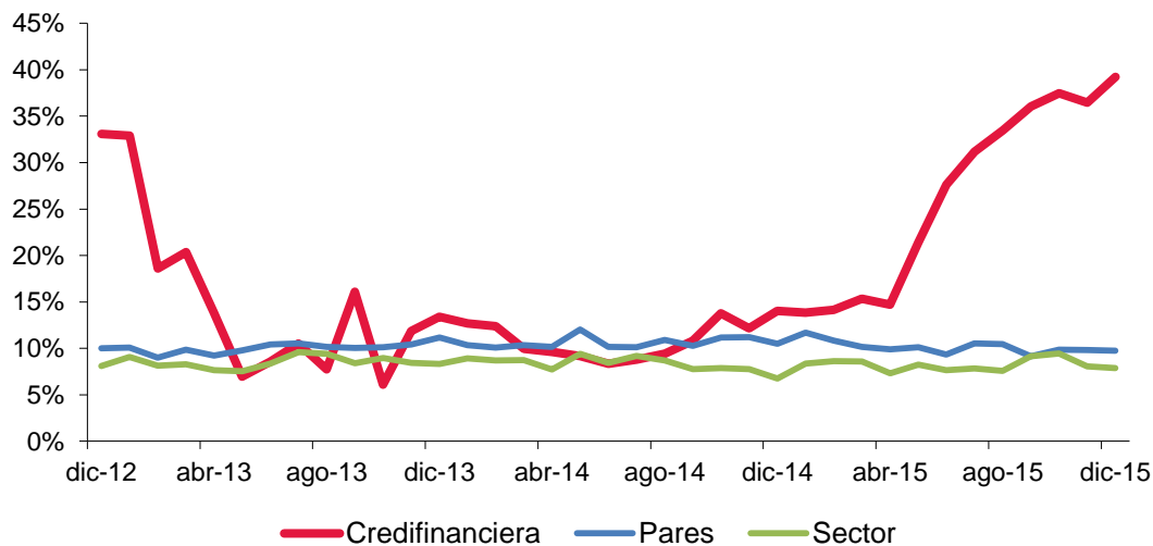
Gráfico 5 Activos líquidos / activos totales
