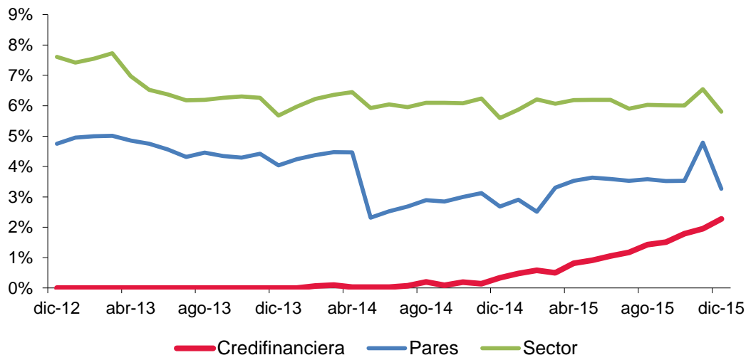
Gráfico 3 Evolución del indicador de calidad de cartera de consumo
